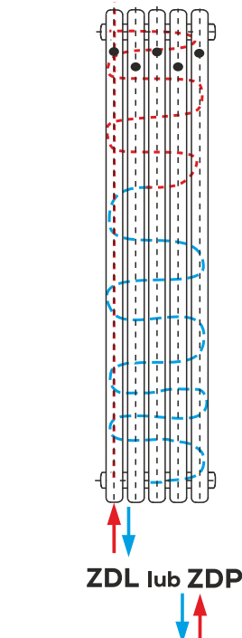
PODŁĄCZENIE DOLNE Z ROZSTAWEM 50 MM
