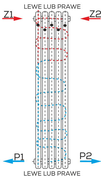
PODŁĄCZENIE STANDARDOWE GÓRA-DÓŁ
