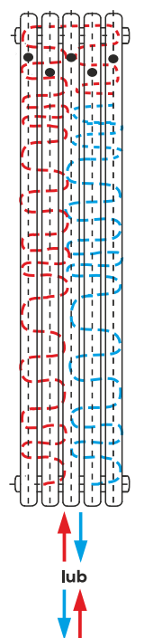
PODŁĄCZENIE DOLNE Z ROZSTAWEM 50 MM
