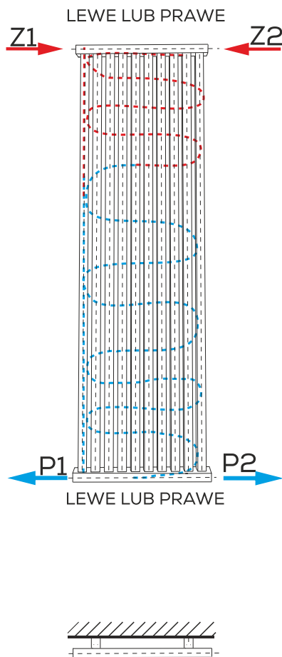
PODŁĄCZENIE STANDARDOWE GÓRA-DÓŁ
