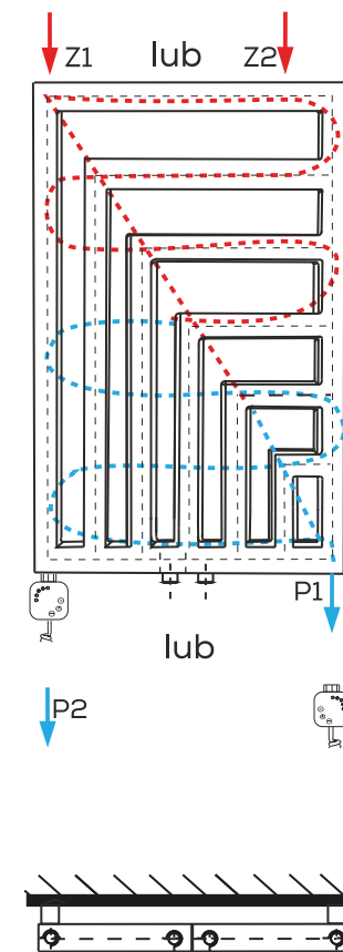
WODNO-ELEKTRYCZNY PODŁĄCZENIE KRZYŻOWE
