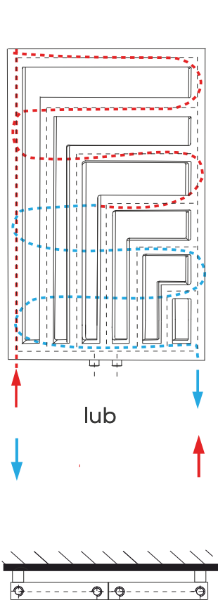
PODŁĄCZENIE OD DOŁU W KOLEKTORACH
