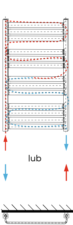
PODŁĄCZENIE OD DOŁU W KOLEKTORACH
