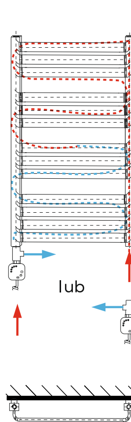
WODNO-ELEKTRYCZNY OD DOŁU W KOLEKTORACH
