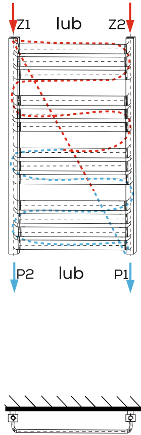
PODŁĄCZENIE KRZYŻOWE
