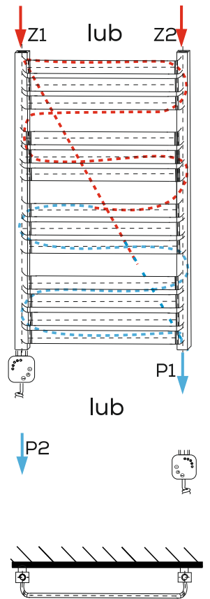
WODNO-ELEKTRYCZNY PODŁĄCZENIE KRZYŻOWE
