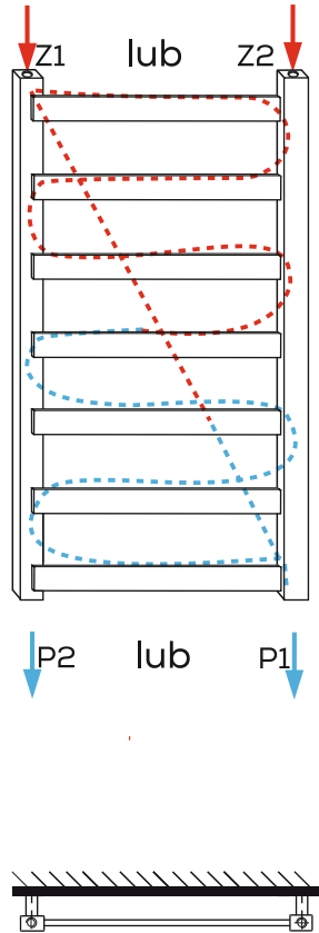
PODŁĄCZENIE KRZYŻOWE
