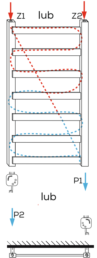
WODNO-ELEKTRYCZNY PODŁĄCZENIE KRZYŻOWE
