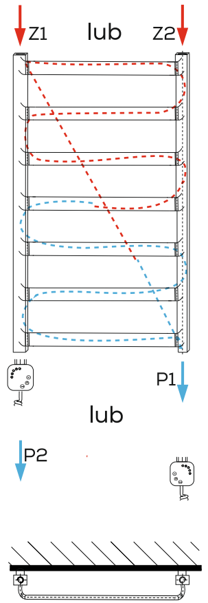
WODNO-ELEKTRYCZNY PODŁĄCZENIE KRZYŻOWE
