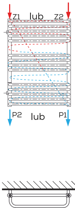
PODŁĄCZENIE KRZYŻOWE
