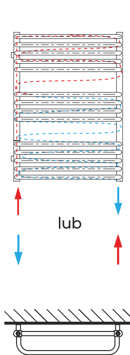
PODŁĄCZENIE OD DOŁU W KOLEKTORACH
