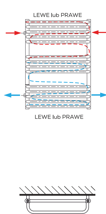
PODŁĄCZENIE BOCZNE
