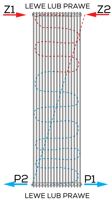
PODŁĄCZENIE KRZYŻOWE
