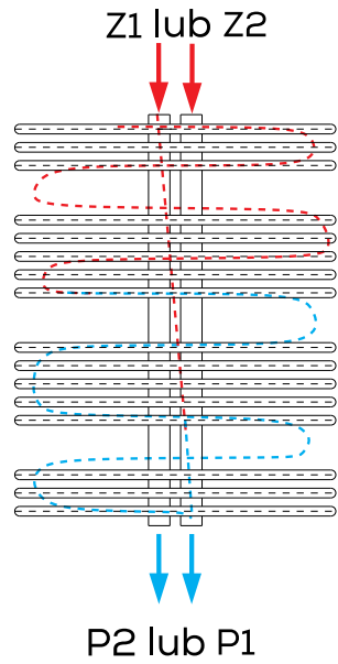
PODŁĄCZENIE KRZYŻOWE
