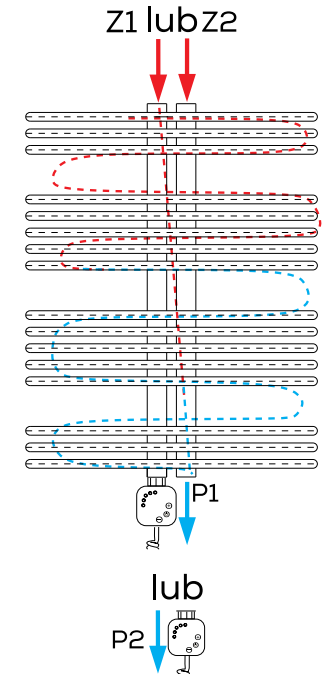
WODNO-ELEKTYCZNY PODŁĄCZENIE KRZYŻOWE
