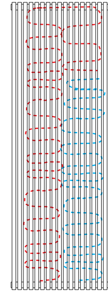
PODŁĄCZENIE DOLNE Z ROZSTAWEM 50 MM
