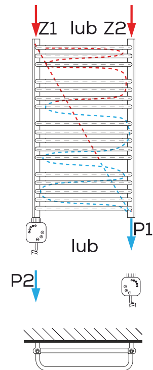
WODNO-ELEKTYCZNY PODŁĄCZENIE KRZYŻOWE
