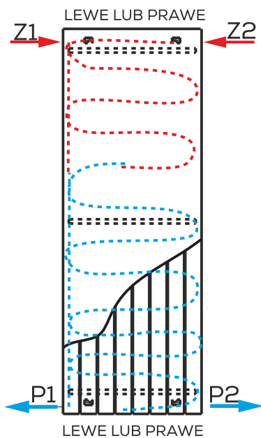
PODŁĄCZENIE STANDARDOWE GÓRA-DÓŁ
