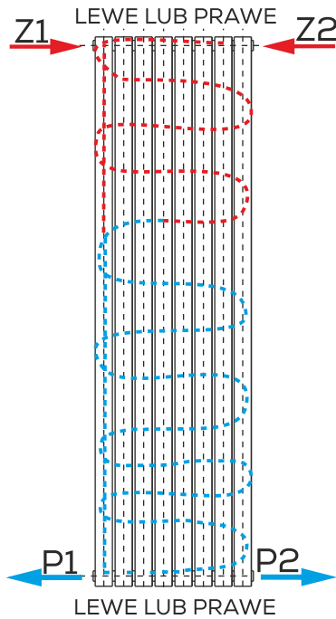
PODŁĄCZENIE STANDARDOWE GÓRA-DÓŁ
