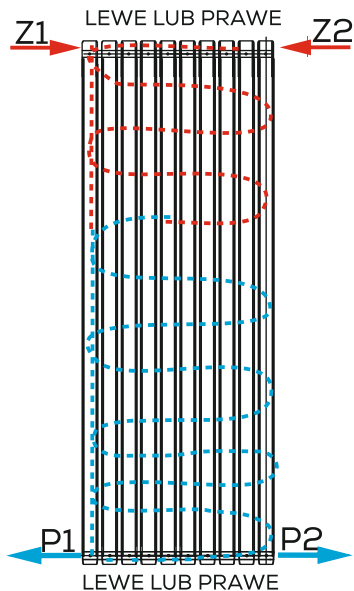
PODŁĄCZENIE STANDARDOWE GÓRA-DÓŁ
