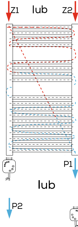
WODNO-ELEKTRYCZNY PODŁĄCZENIE KRZYŻOWE
