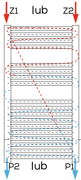
PODŁĄCZENIE KRZYŻOWE
