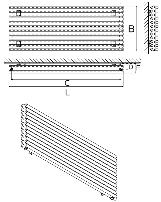
Wersja pozioma w standardzie z zasileniem dolnym w kolektorach
