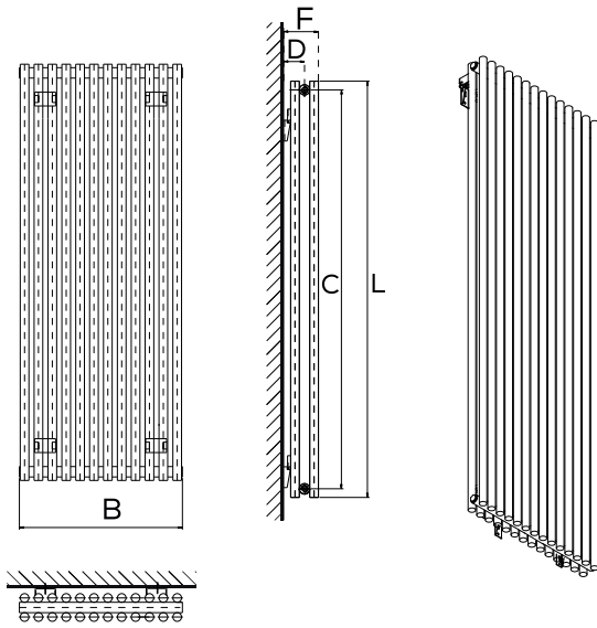
Wersja standardowa w pionie z zasileniem bocznym w kolektorach
