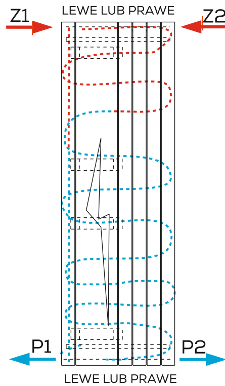
PODŁĄCZENIE STANDARDOWE GÓRA-DÓŁ
