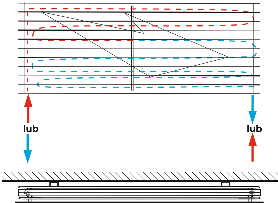
STANDARDOWE PODŁĄCZENIE OD DOŁU W KOLEKTORACH PO SZEROKOŚCI GRZEJNIKA
