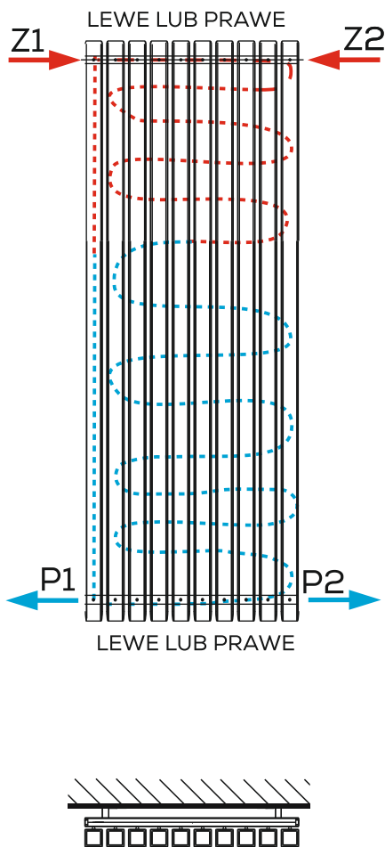
PODŁĄCZENIE STANDARDOWE GÓRA-DÓŁ
