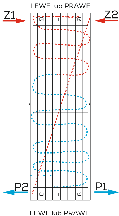
PODŁĄCZENIE KRZYŻOWE
