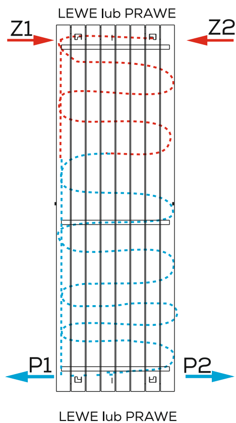
PODŁĄCZENIE STANDARDOWE GÓRA-DÓŁ
