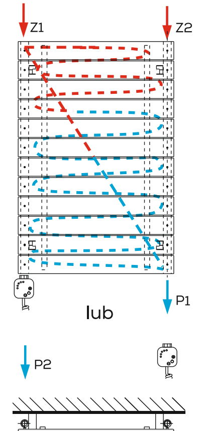
WODNO-ELEKTRYCZNY PODŁĄCZENIE KRZYŻOWE
