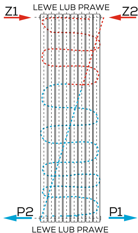
PODŁĄCZENIE KRZYŻOWE
