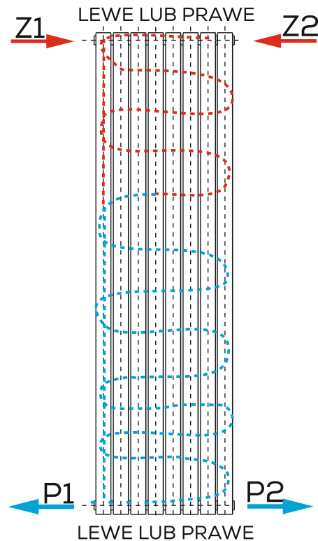
PODŁĄCZENIE STANDARDOWE GÓRA-DÓŁ
