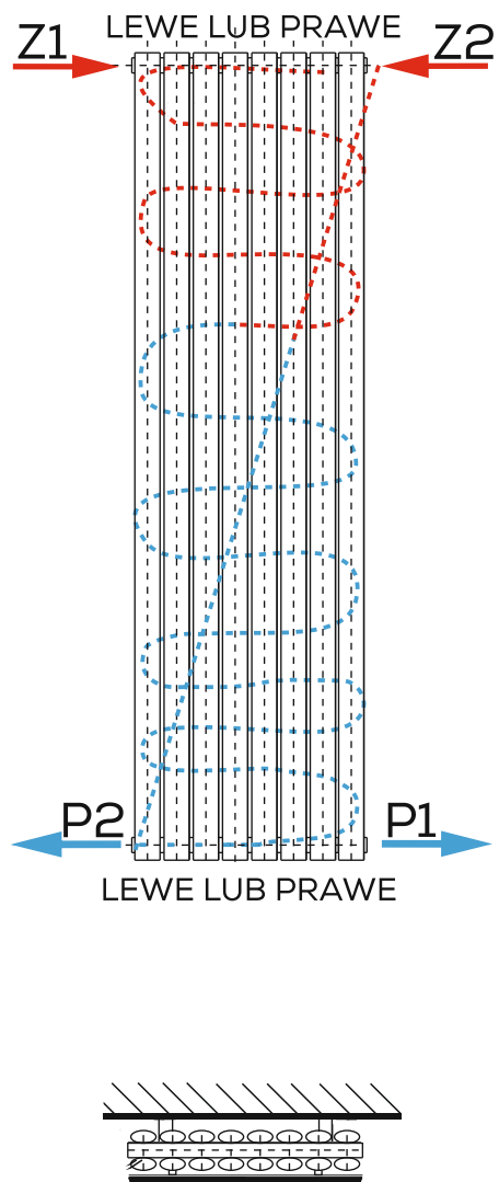
PODŁĄCZENIE KRZYŻOWE
