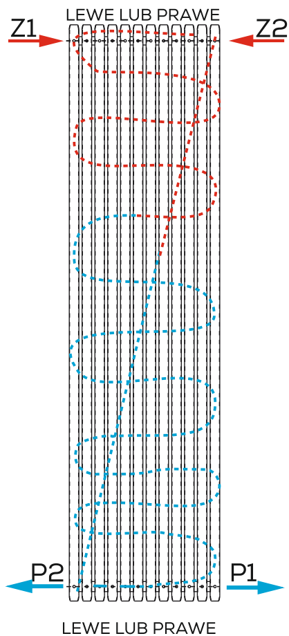
PODŁĄCZENIE KRZYŻOWE
