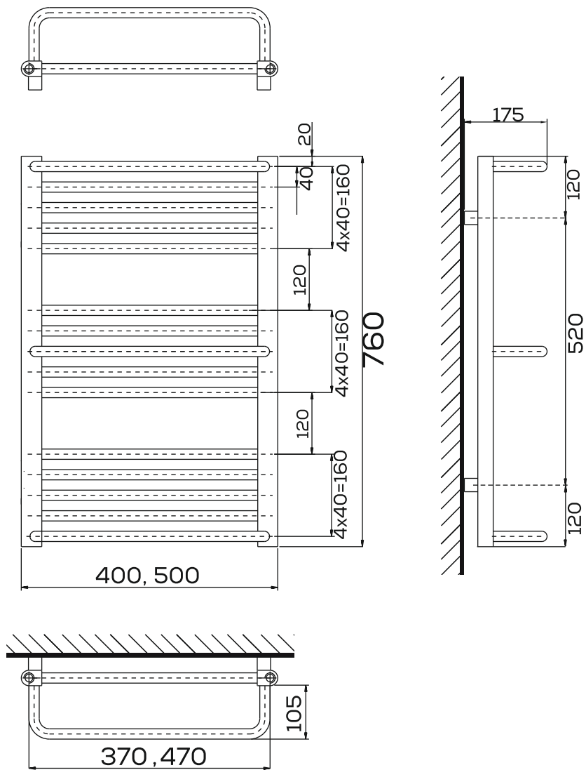
GRZEJNIK Z PODŁĄCZENIEM DOLNYM W KOLEKTORACH
