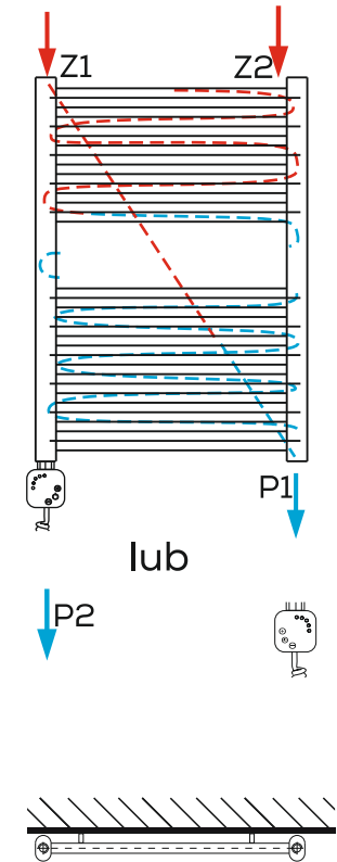
WODNO-ELEKTRYCZNY PODŁĄCZENIE KRZYŻOWE
