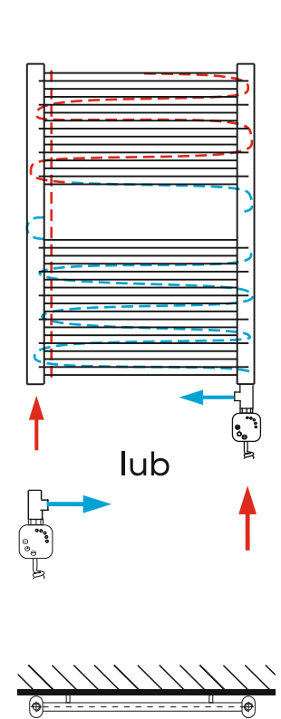
WODNO-ELEKTRYCZNY OD DOŁU W KOLEKTORACH
